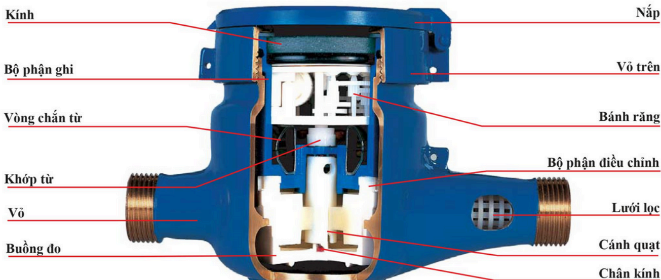
Mặt cắt của đồng hồ đo nước Thái Aichi loại MAM
